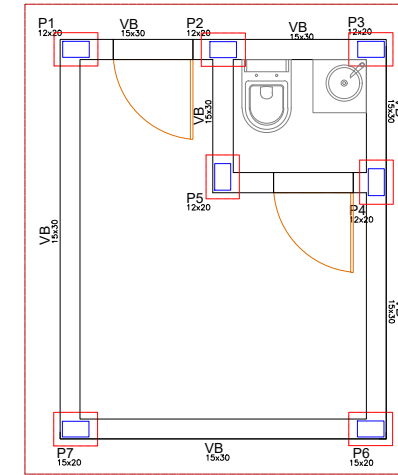
ESTRUTURAL - BALDRAME
